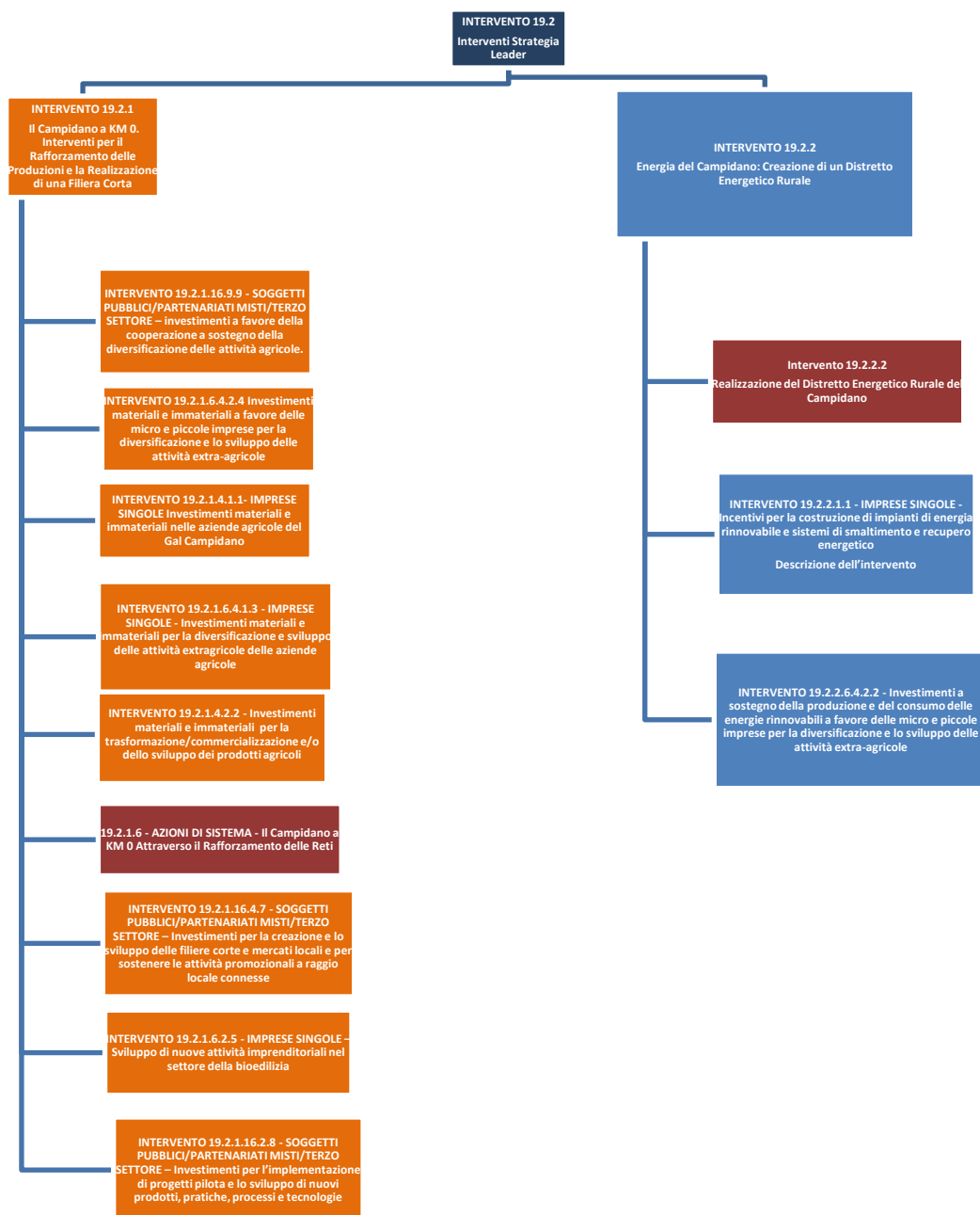
Figura 1. La gerarchia tra operazioni
